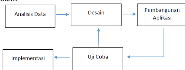
Gambar 1. Prosedur Pengembangan
