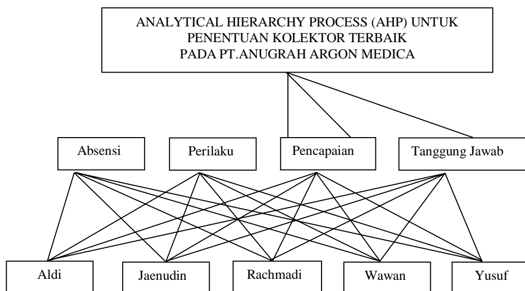
Gambar 1. Struktur Hirarki
